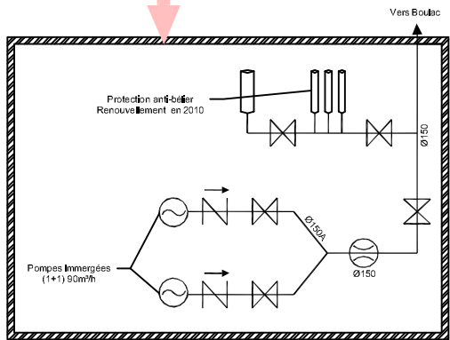
Zoom de la chambre de vannes
